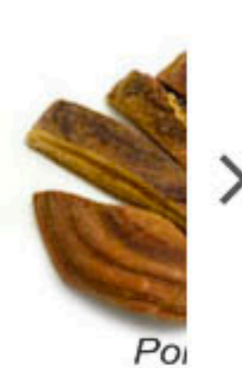
Poria
